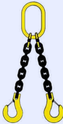
Ref FC-LCO2-ASF/GCT
