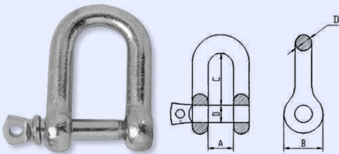
Manilha Retas Padrão - Fator de Segurança 4:1
