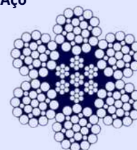
6x25 Filler 1+6+6+12
