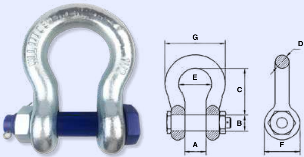
Manilha Curva com Pino Porca e Cupilha (G2130) - Fator de Segurança 6:1
