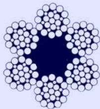
6x25 Filler 1+6+6+12
